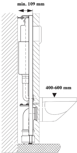
Ohut elementti lattiaviemäroinnilla
