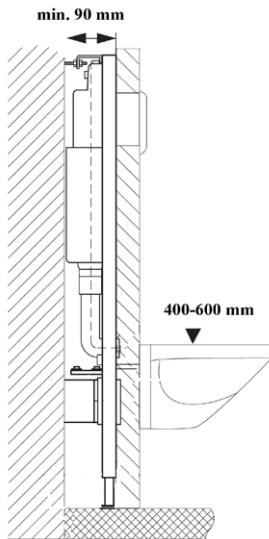
Ohut elementti seinäviemäroinnilla
